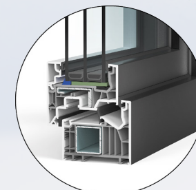
Flächenversetzte Variante
