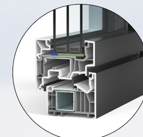
Flächenbündige Variante
